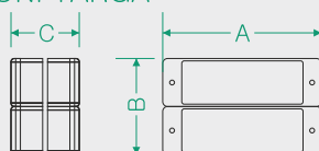
DIMENSIONI TARGA
